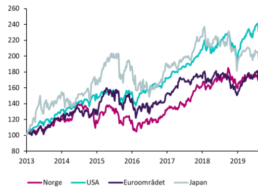
Figur 2.2. Aksjekurser. Indeks
